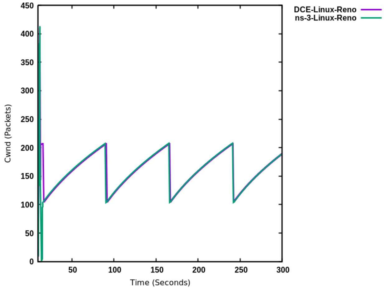
Fig. 9: DCE Linux Reno vs. ns-3 Linux Reno
